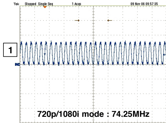
< VOUT_CLK >
