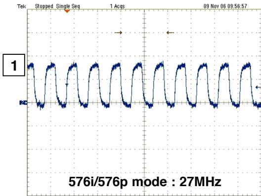
< VOUT_CLK >
